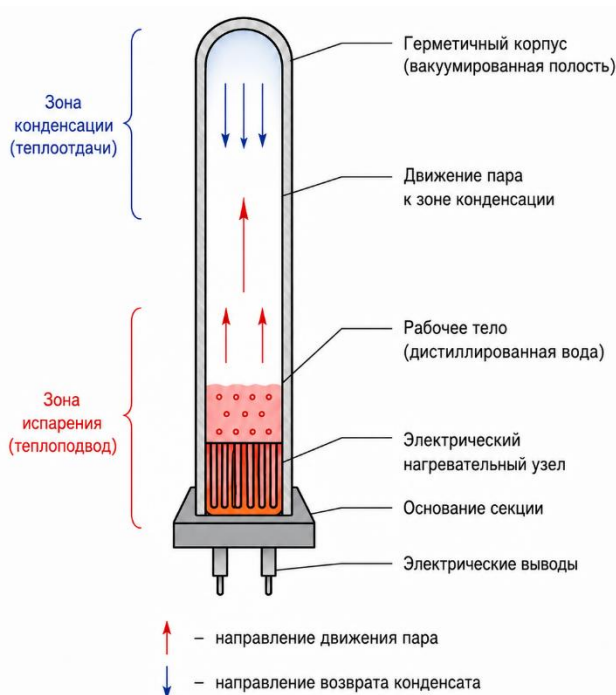
Рисунок 1.3 – Принципиальная схема секции ПЭНД на основе ЭВТТ гравитационного типа
