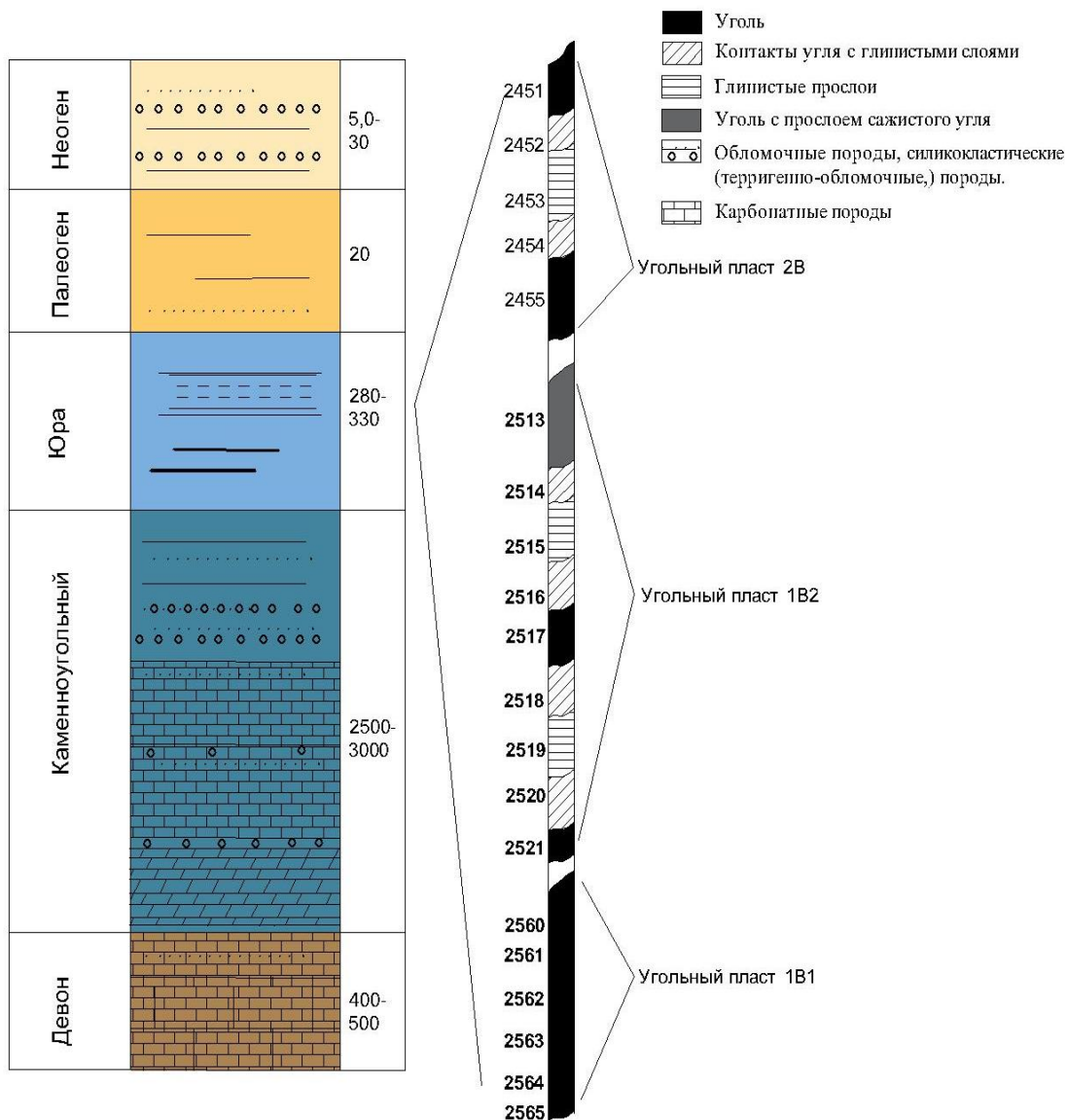
Рисунок 2.1 – Геологическая позиция угольных пластов на месторождении Шубарколь
