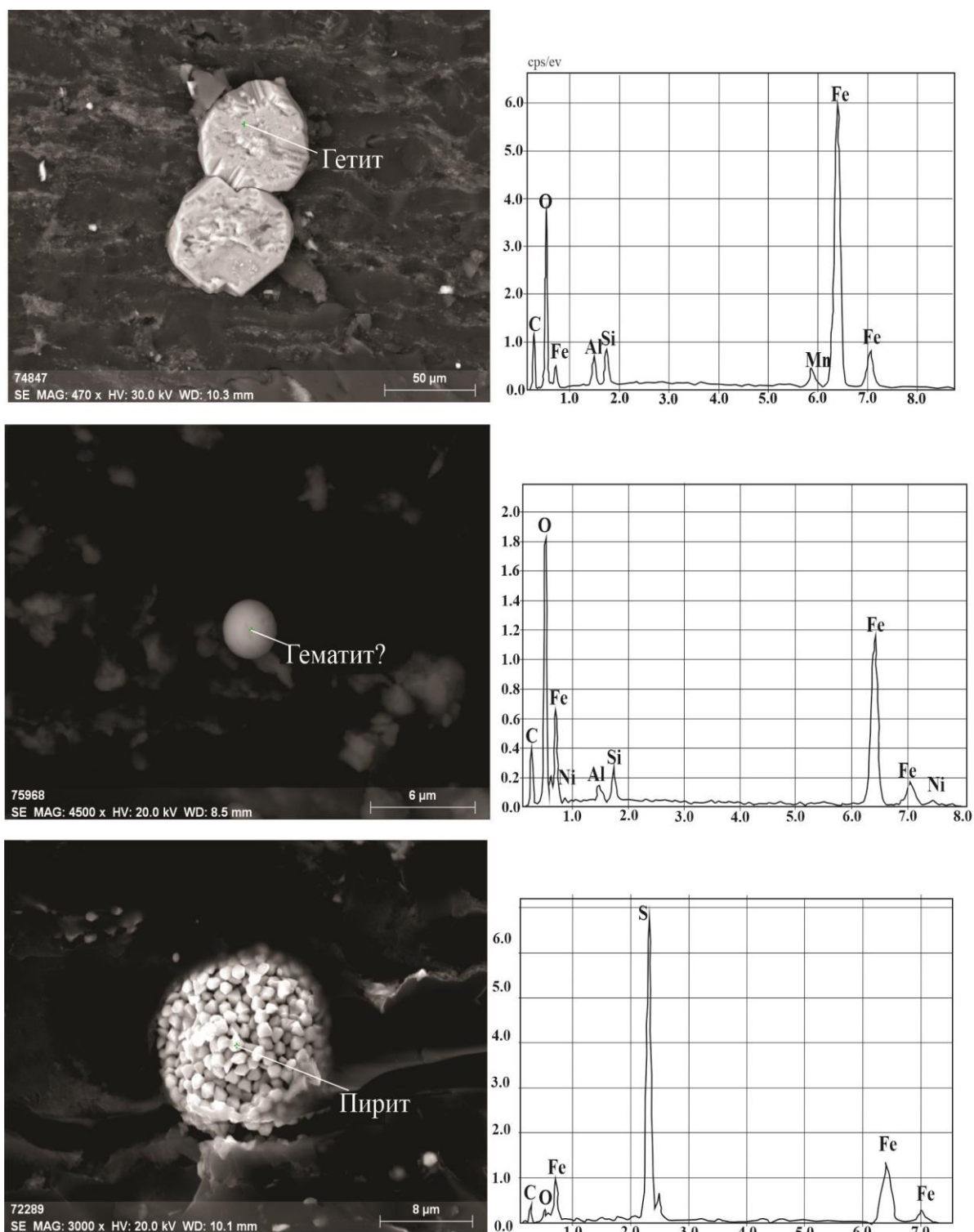
Рисунок 5.9 – Оксиды железа (вверху и в середине) и фрамбоидальный пирит (внизу) На нижнем рисунке это пирит, на верхнем – это гетит, гематит, на среднем – возможно, это космическая микросфера гетита, гематита или магнетита?
