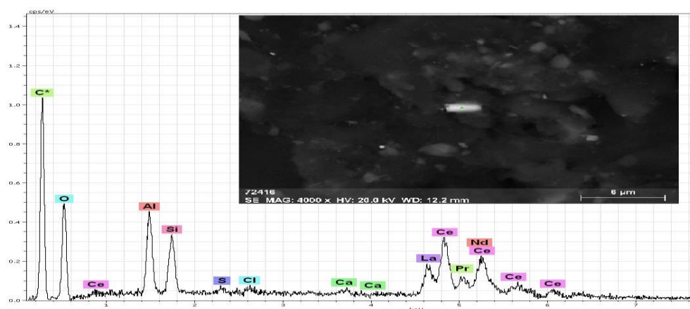
Рисунок 5.6 – Бастензит?
