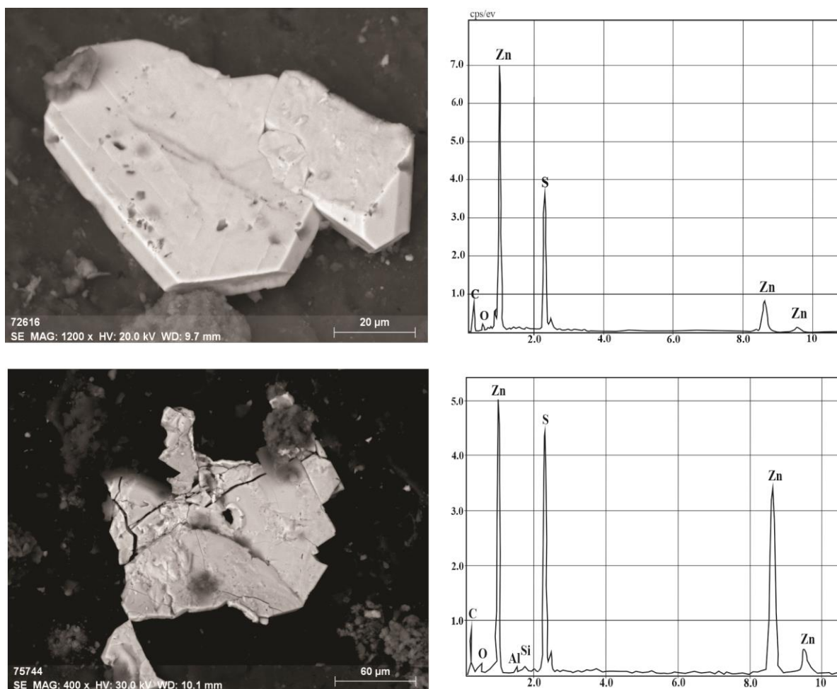
Рисунок 5.13 – Сфалерит
