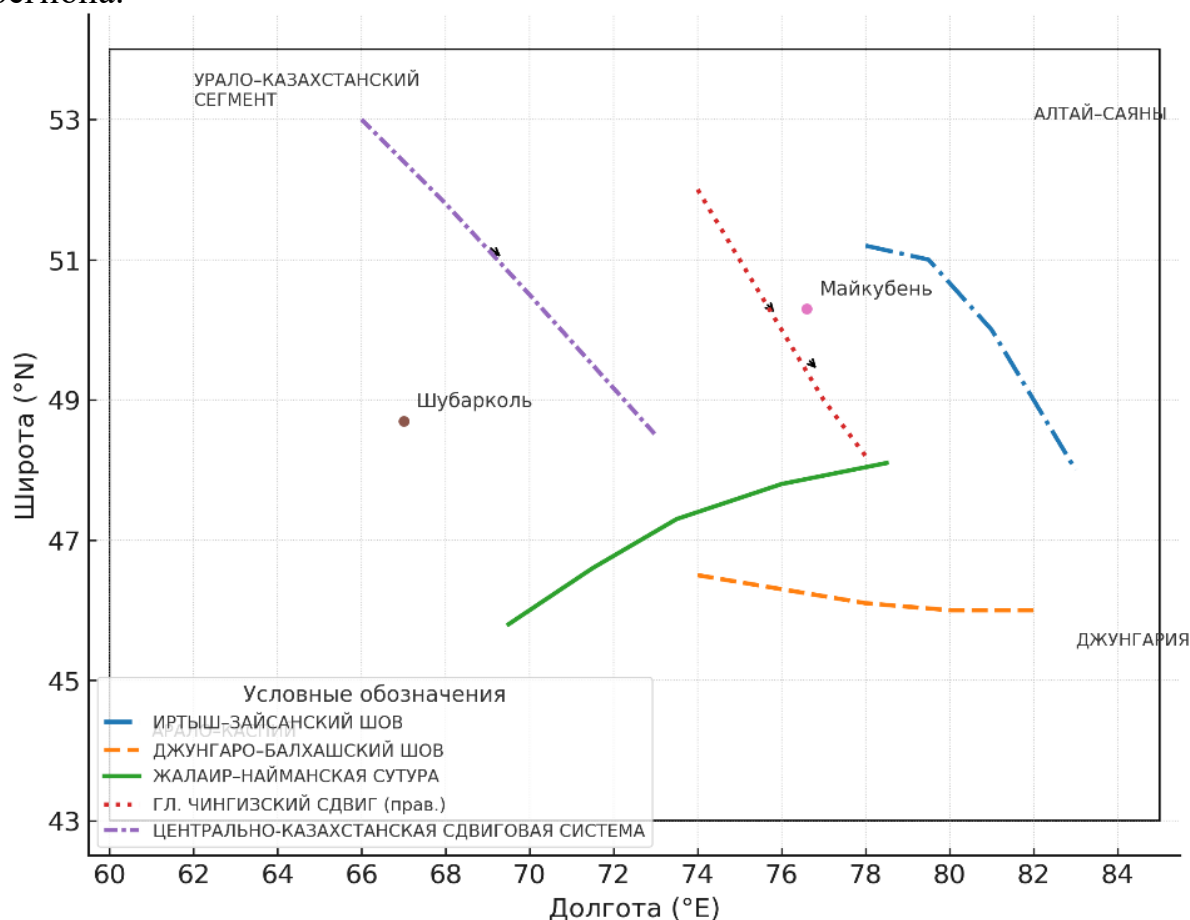
Рисунок 3.2 – Положение Майкубеньского бассейна и месторождения Шубаркуль в системе геодинамических структур западной части Центрально-Азиатского орогенного пояса [составлена автором по данным 38, 41, 46, 47, 48]
