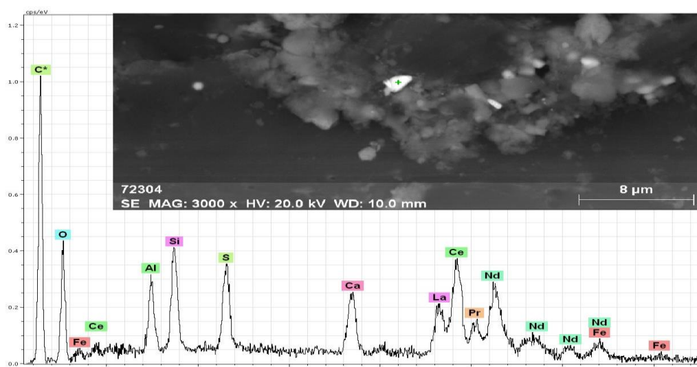
Рисунок 5.5 – Монацит
