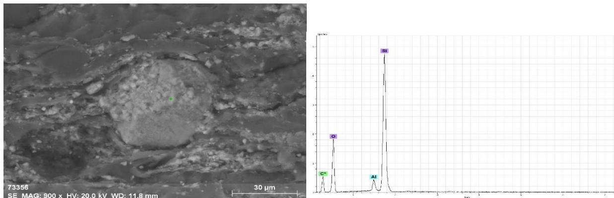
Рисунок 5.1 – Кварц
