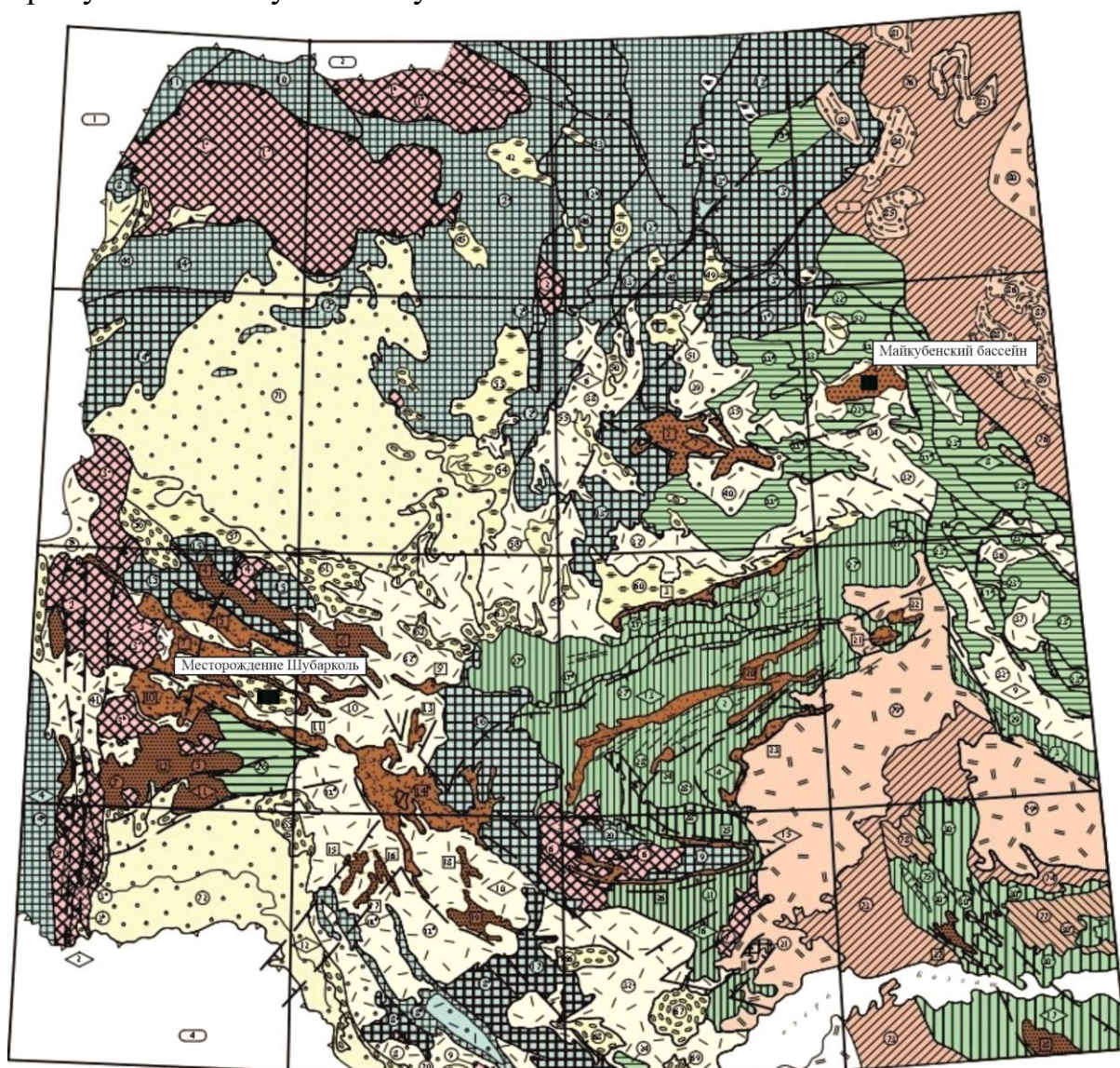
Рисунок 3.3 – Схема основных структур Центрального Казахстана [50]
