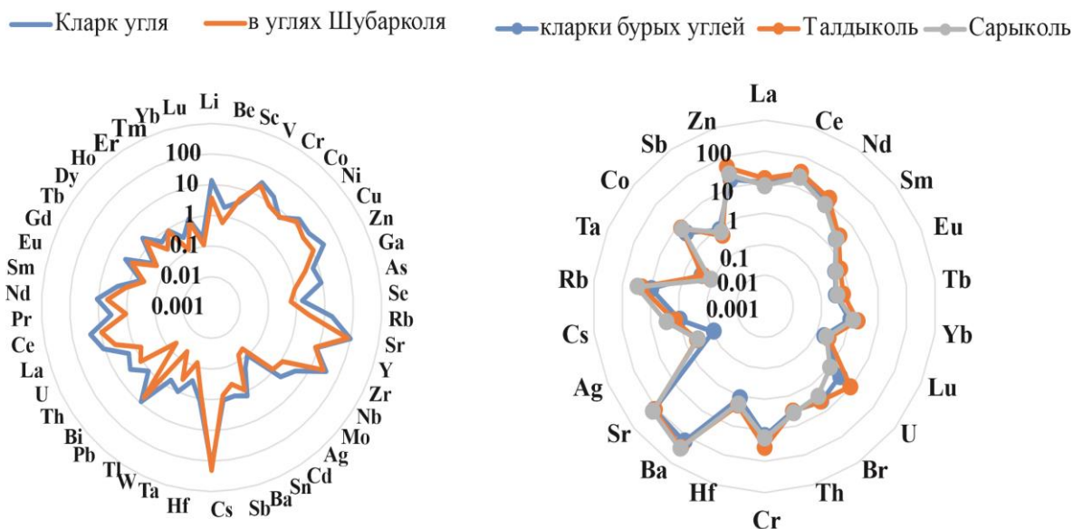
Рисунок 4.1 – Сравнение среднего содержания элементов-примесей и РЗЭ в углях а) месторождения Шубарколь с кларками для каменных углей, б) бассейна Майкубень с кларками для бурых углей [81]
