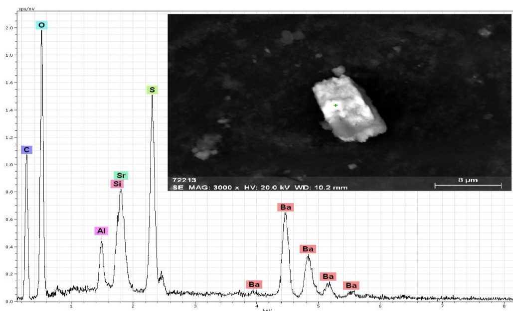
Рисунок 5.16 – Частицы целестина \text{SrSO}_4 с включениями Ba
