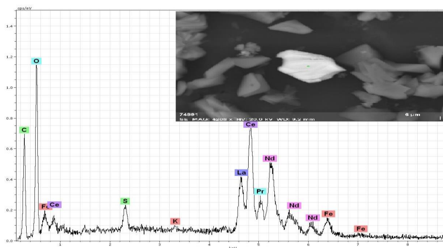
Рисунок 5.7 – Оксид (карбонат) редкоземельных элементов
