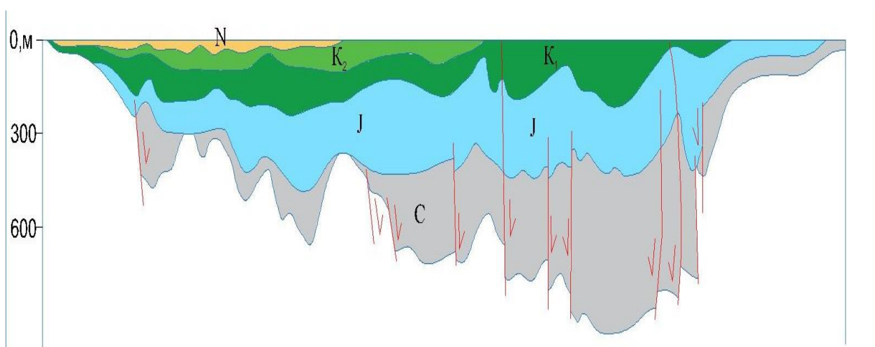
Рисунок 3.6 – Поперечный разрез типичного внутриконтинентального бассейна растяжения (изменено из [53])
