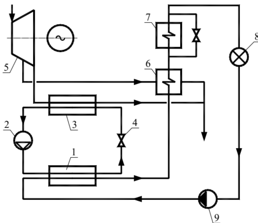
Рисунок 1 - Схема использования ТНУ в качестве подогревателя нижней ступени сетевого подогрева на ТЭЦ: 1 – конденсатор; 2 – компрессор; 3 – испаритель; 4 – дроссель; 5 – турбина; 6 – сетевой подогреватель; 7 – пиковый водогрейный котел; 8 – потребитель; 9 – сетевой насос
