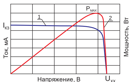
Рисунок 2 - Вольт-амперная (1) и Ватт-амперная (2) характеристики солнечной панели
