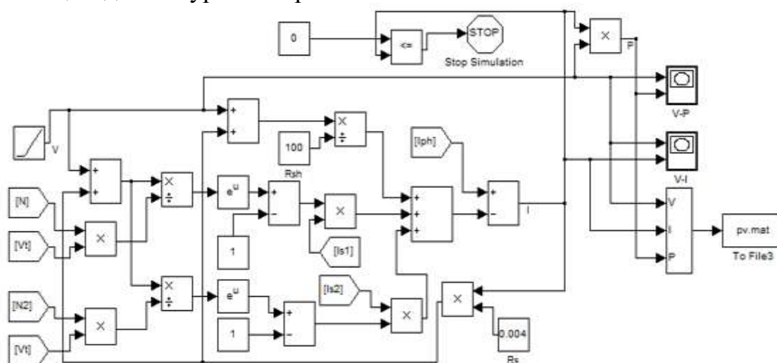
Сурет 2 - Simulink бағдарламасында жүзеге асырылған гибридті күн энергиясын түрлендіру жүйесінің моделі
