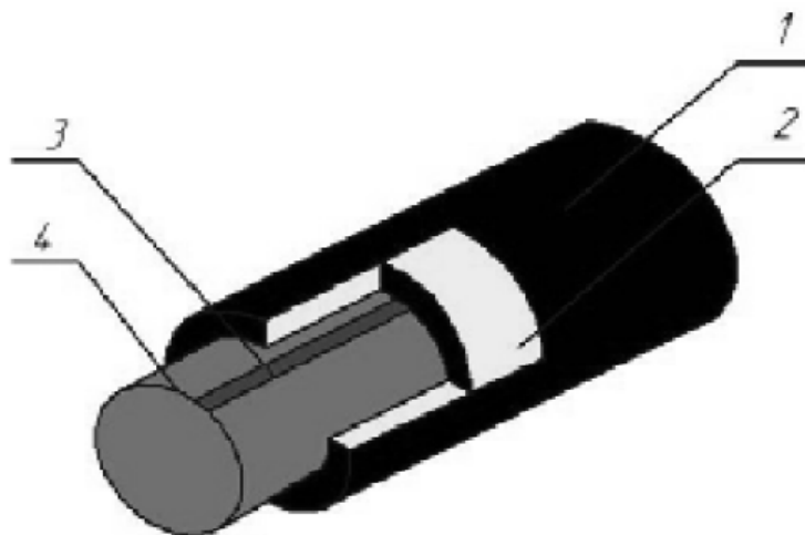
Сур. 1. Алдын ала оқшауланған құбыр ППУ бөлінісінде: 1-құбыр қабықша; 2 – изоляция из ППУ; 3-болат құбыр; 4 – сигналдық сым жүйесін ББК
