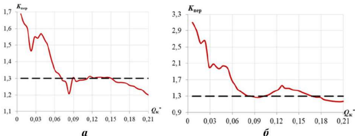
Рисунок 2 - Зависимость коэффициента перегрузки K_{пер} от мощности батареи конденсаторов: а – физическая модель, б – компьютерная модель
