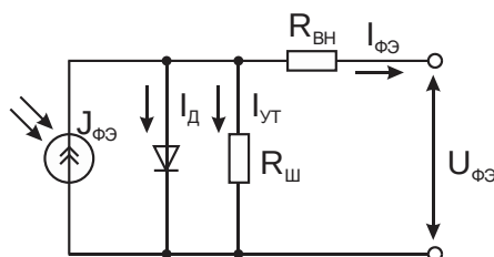
Рисунок 3 – Упрощенная схема замещения ячейки солнечной панели
