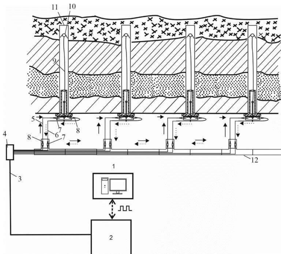
Рисунок 1 – Конструкция системы
