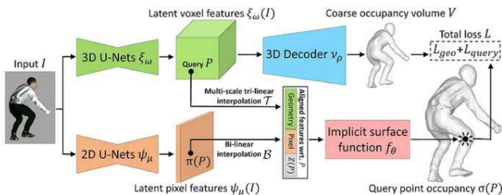
Рисунок 3 – Алгоритм работы нейронных сетей
