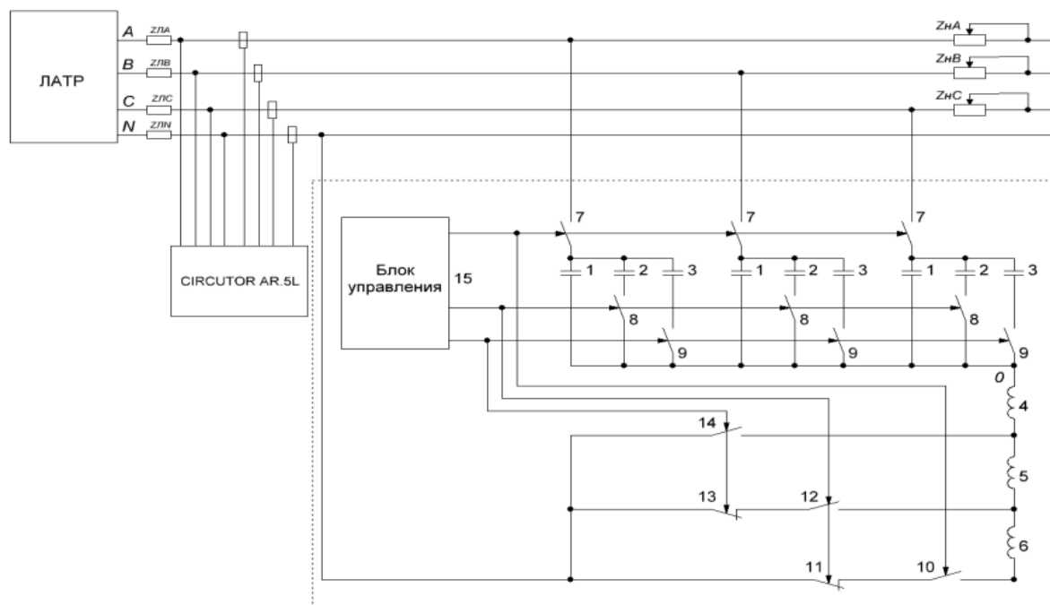
Рисунок 1 - Электрическая схема экспериментальной установки: 1-3 – емкостные элементы; 4-6 – реакторы; 7-10, 12, 14 – замыкающие контакты; 11, 13 – размыкающие контакты; 15 – блок управления
