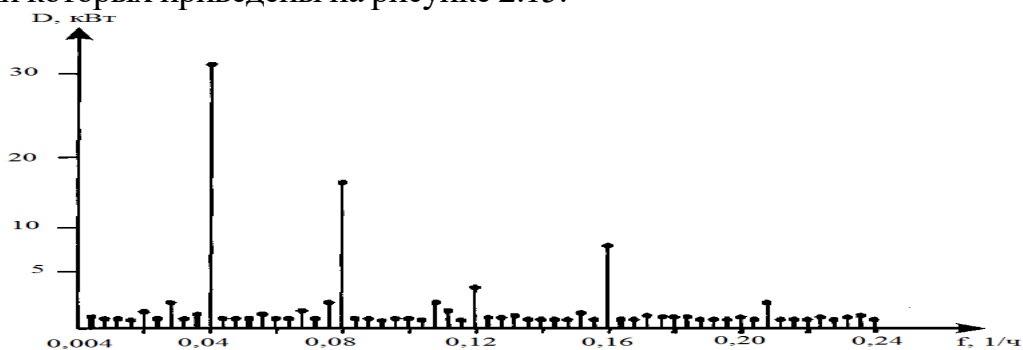
Рисунок 2.15 - Дисперсионный спектр подземной нагрузки
