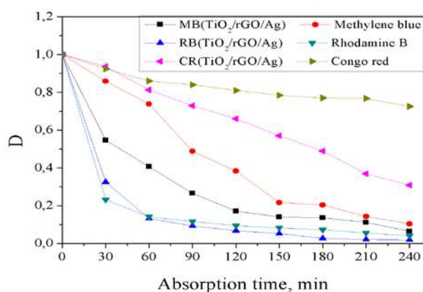
Сурет 2. \text{TiO}_2/\text{rGO}/\text{Ag} MB, Rh B, CR бояғыш ерітінділеріндегі ыдырау процесі
