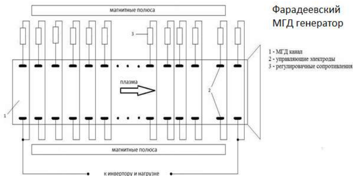
Рис. 1. Схема фарадеевского МГД генератора
