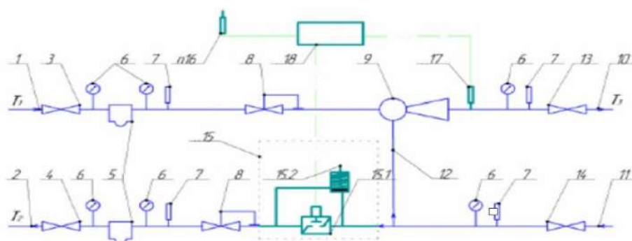
Рисунок 1 – Схема элеваторного узла с импульсным подмесом теплоносителя
