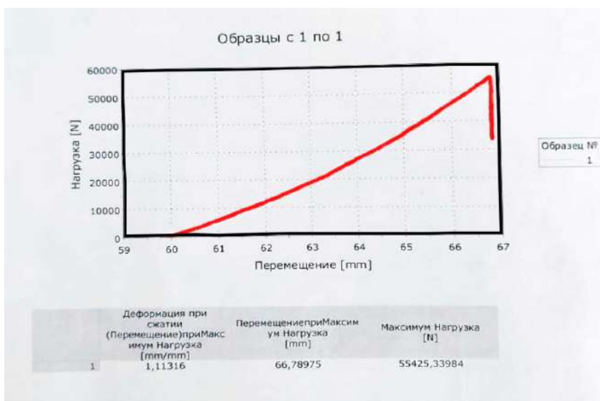
Рисунок 1 - График зависимости нагрузки от перемещения для направляющего устройства d=80\text{мм}
