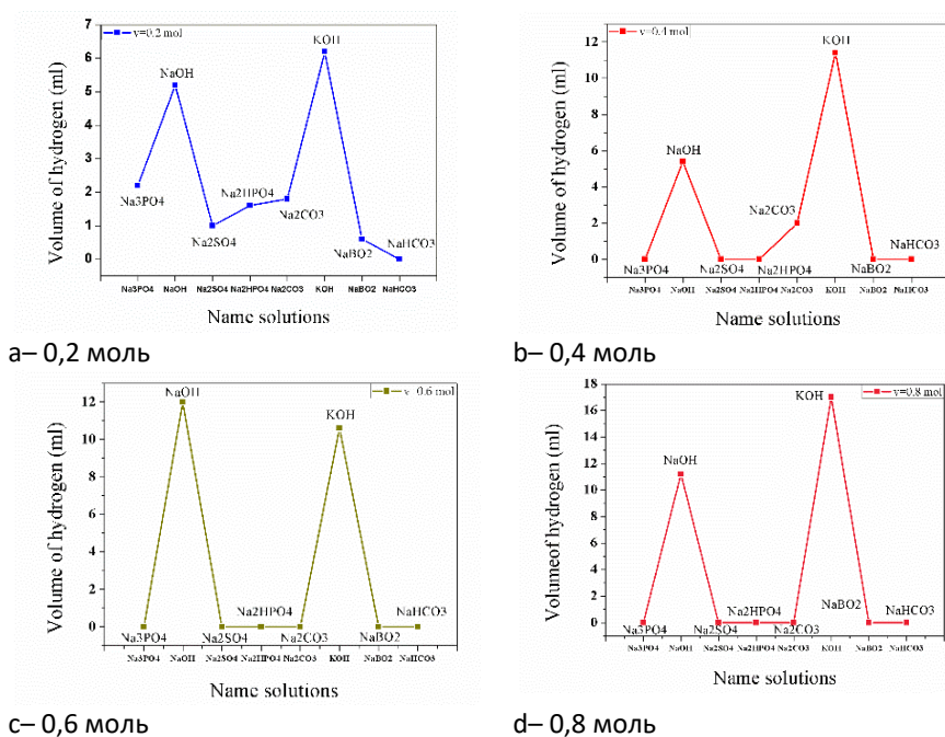
1-сурет. Судың ыдырау процесіне ерітінділердің әсері
