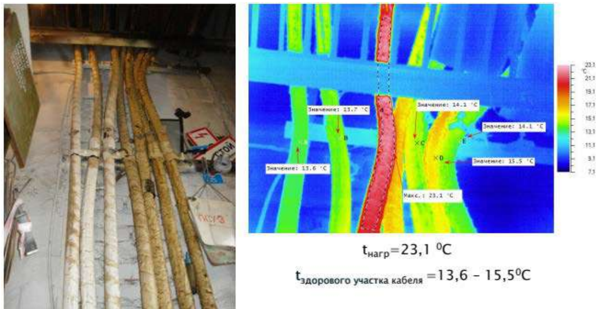
Рисунок 2 - Нагрев участка кабеля от концевой муфты до входа в кабельный тоннель вследствие осушения
