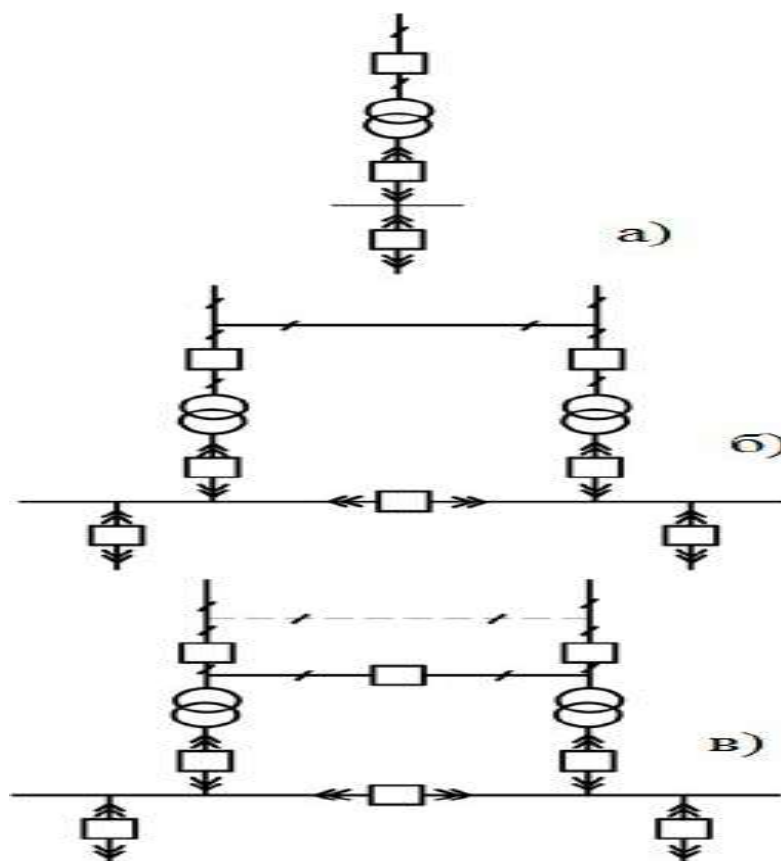
Рисунок 3 – Типовые схемы подстанций
