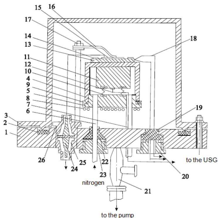
1-сурет. Поляризацияның, поляризацияның термоинтандырылған токтарын және диэлектрлік шығын бұрышының тангенсін өлшеуге арналған қондырғының конструкциясы
