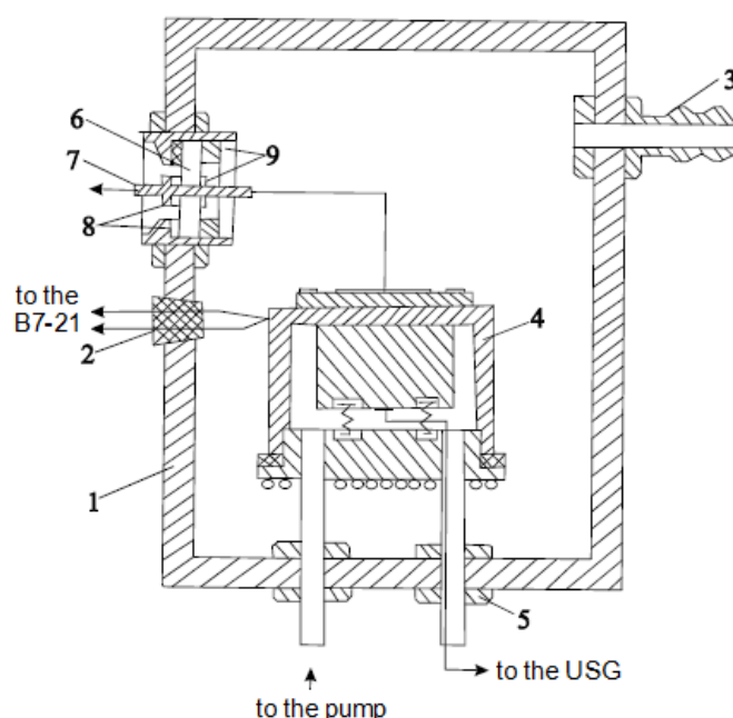
2-сурет. \text{tg}\delta және \epsilon' шағын мәндерін өлшеуге арналған қондырғының конструкциясы
