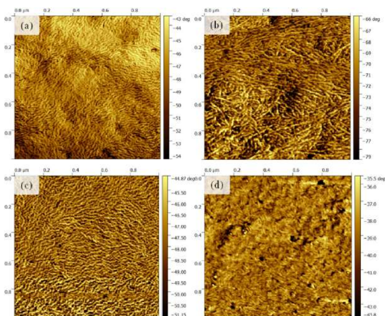
Fig.1. AFM phase contrast images of a) P3HT, b) \text{MoS}_2 -NP P3HT, c) P3HT:PC61BM, d) \text{MoS}_2 -NP P3HT:PC61BM
