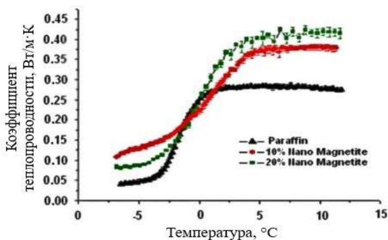
Рисунок 1 – График зависимости коэффициента теплопроводности материалов от температуры
