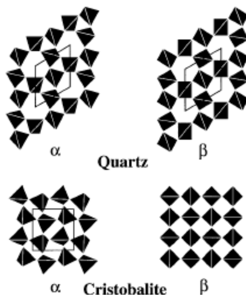
Рисунок 1. Сравнение структур кварца и кристобалита.
