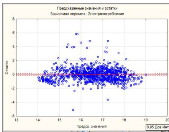
Рисунок 3 – Предсказанные значения и остатки
