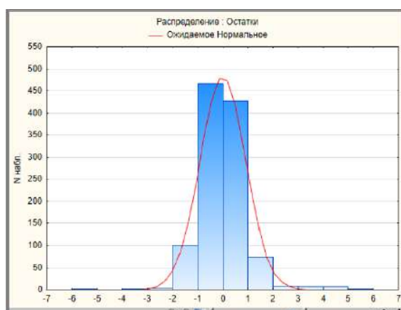
Рисунок 1 – Гистограмма распределения остатков
