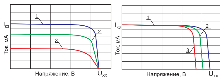
а) 1 – 1000 Вт/м 2 ; 2 – 600 Вт/м 2 ; 3 – 400 Вт/м 2 б) 1 – 0 °C; 2 – 20 °C; 3 – 40 °C
