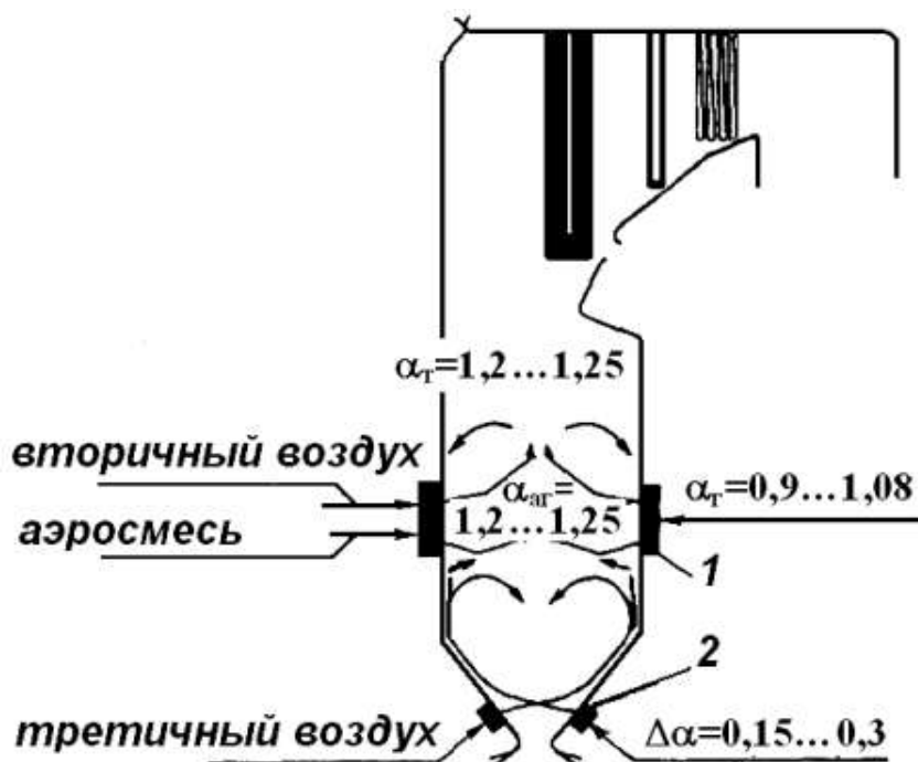
Рисунок 1 - Схема топочно-горелочного устройства с нижним дутьем: 1 - горелка; 2 - сопло нижнего дутья.
