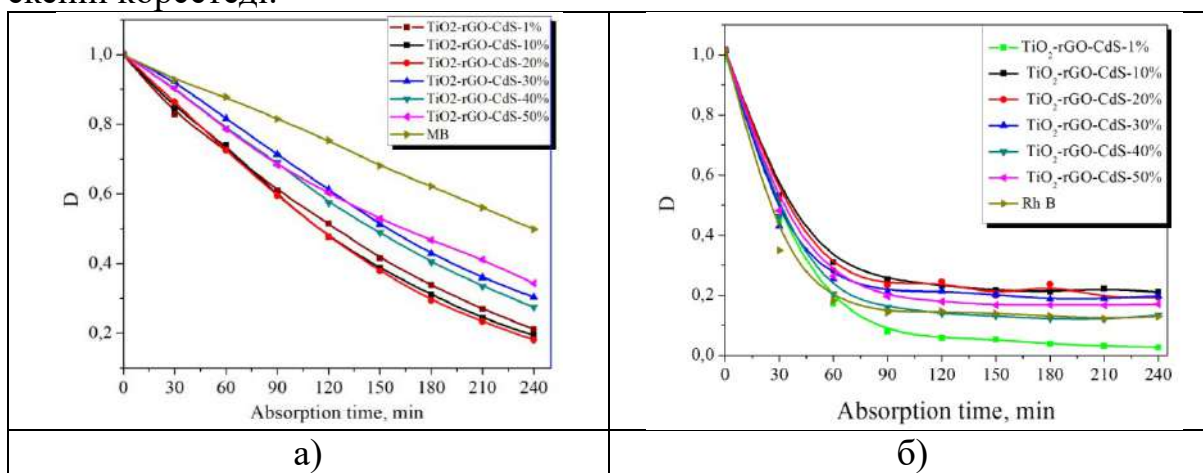
Сурет 2. \text{TiO}_2/\text{rGO}/\text{CdS} нанокөмбірі үшін MB, RhB ыдырау процесі
