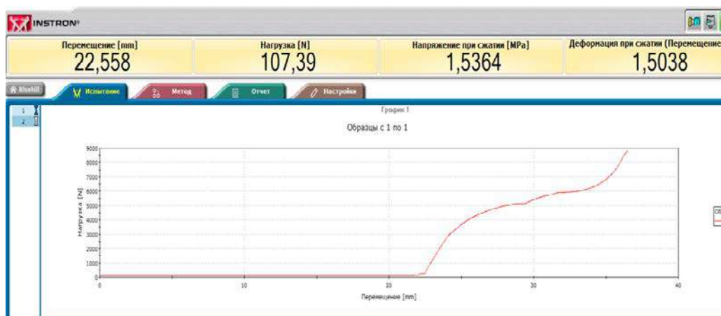
Рисунок 2 - График зависимости нагрузки от перемещения для направляющего устройства d=50\text{мм}
