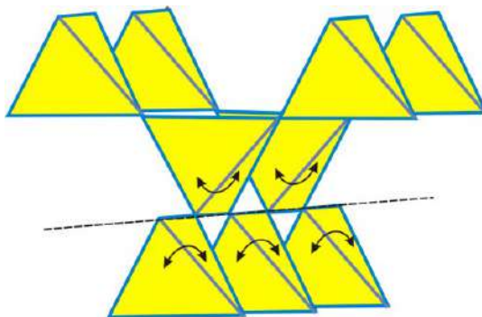
Рисунок 3. Линейные цепочки, проходящие через один из тетраэдров в структуре кристобалита.
