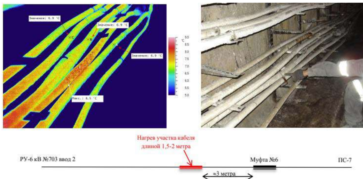
Рисунок 1 - Нагрев участка изоляции кабеля, t_{\text{нагр}} = 8,5^{\circ}\text{C} , t_{\text{здорового участка кабеля}} = 6,9^{\circ}\text{C}
