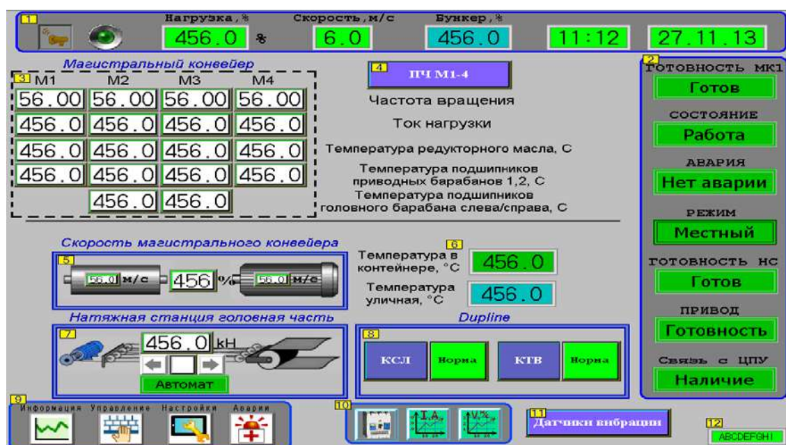
Рисунок 1 – Основной экран
