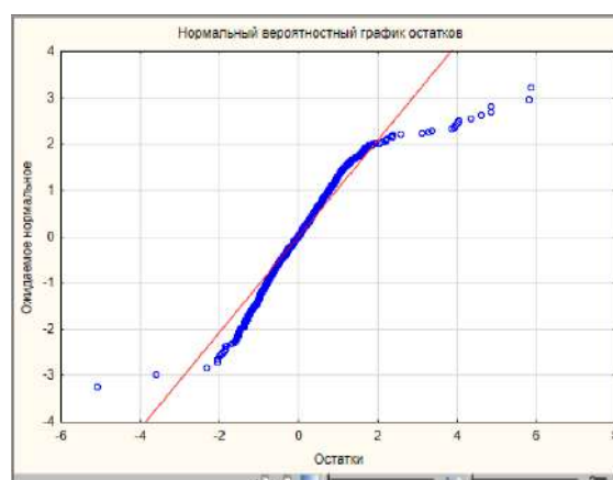
Рисунок 2 – Нормальный вероятностный график остатков
