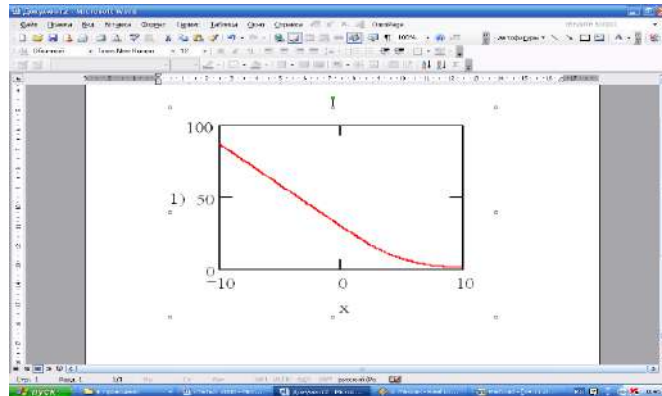
Рис.1. Решение однородной задачи теплопроводности
