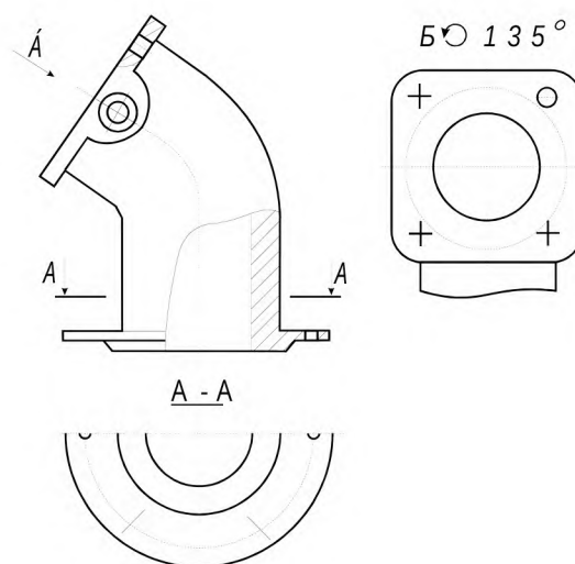
Рисунок 5.2 – Изображение на чертежах дополнительных видов
