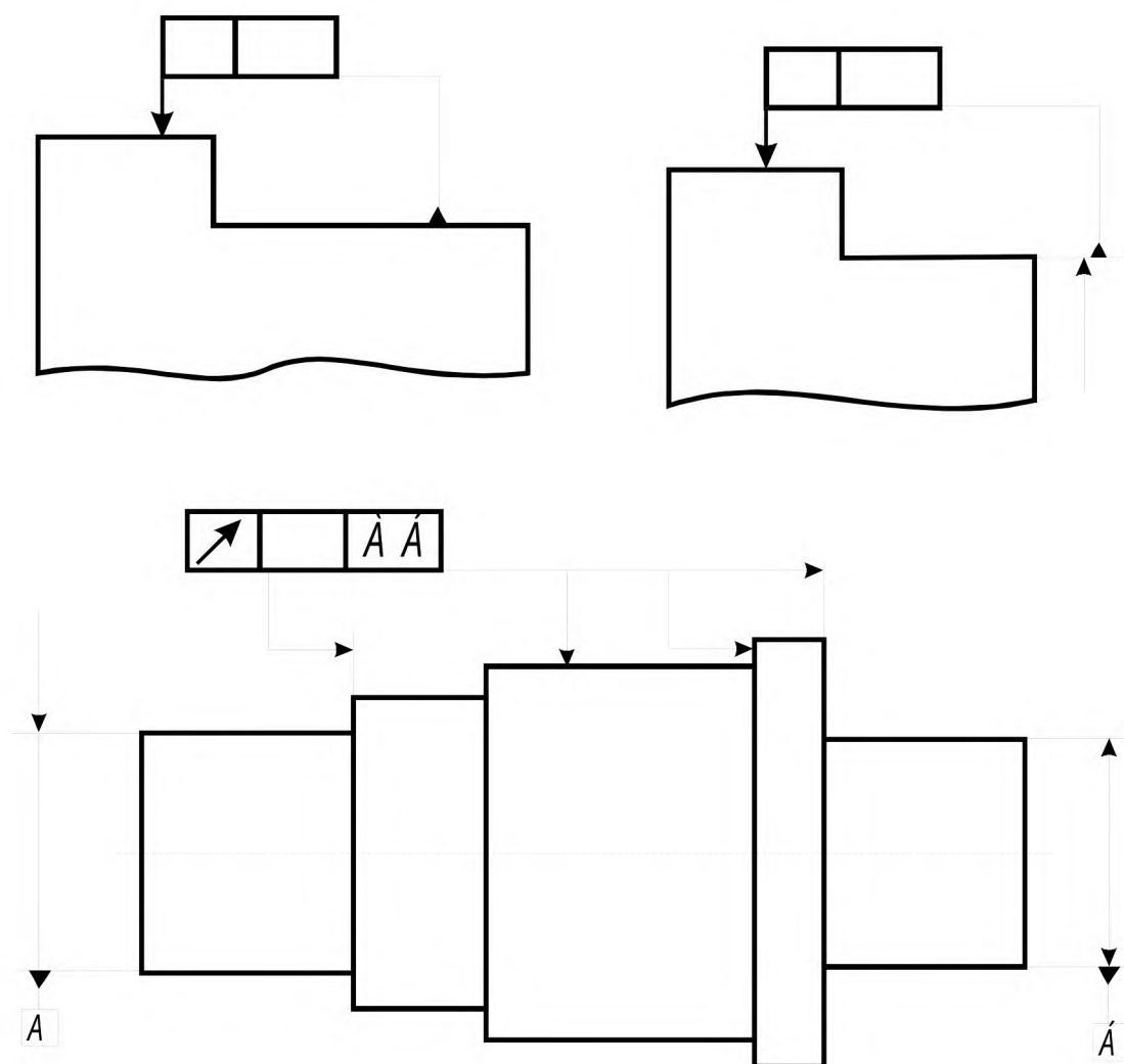
Рисунок 5.12 – Обозначение баз на чертежах
