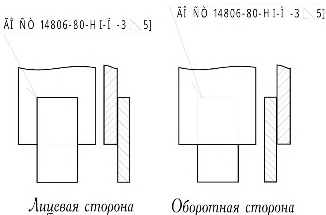
Рисунок 5.20 – Примеры условного обозначения сварных швов на чертежах
