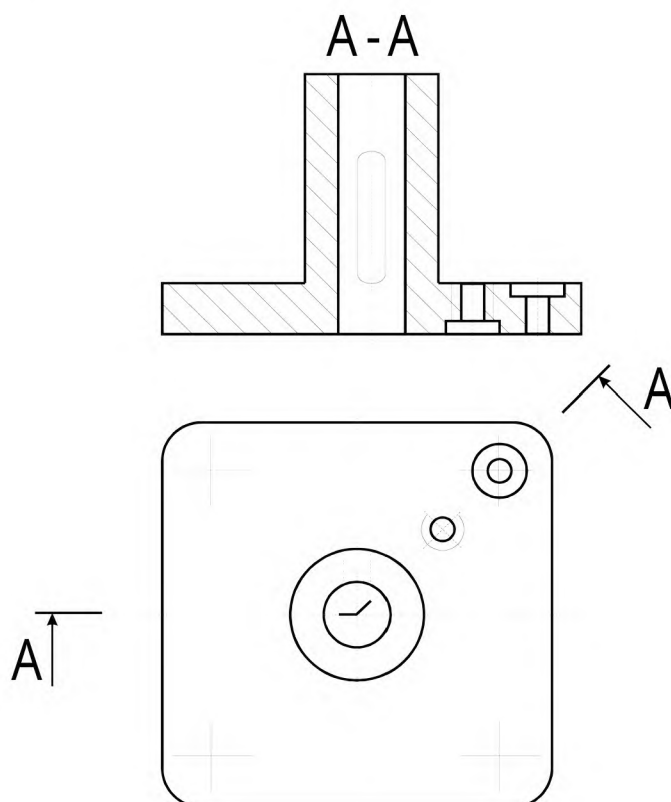
Рисунок 5.4 – Изображение разрезов и секущей линии на чертежах
