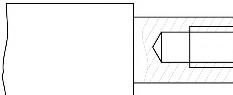
Рисунок 5.5 – Изображение на чертеже местного разреза
