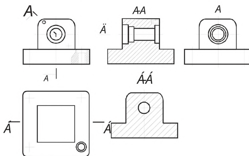
Рисунок 5.1 – Изображение на чертежах видов или разрезов не связанных проекционно с главным изображением
