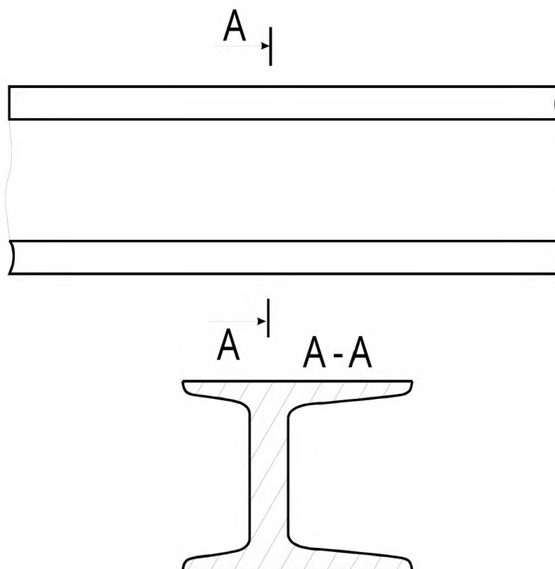
Рисунок 5.6 – Вынесенные сечения
