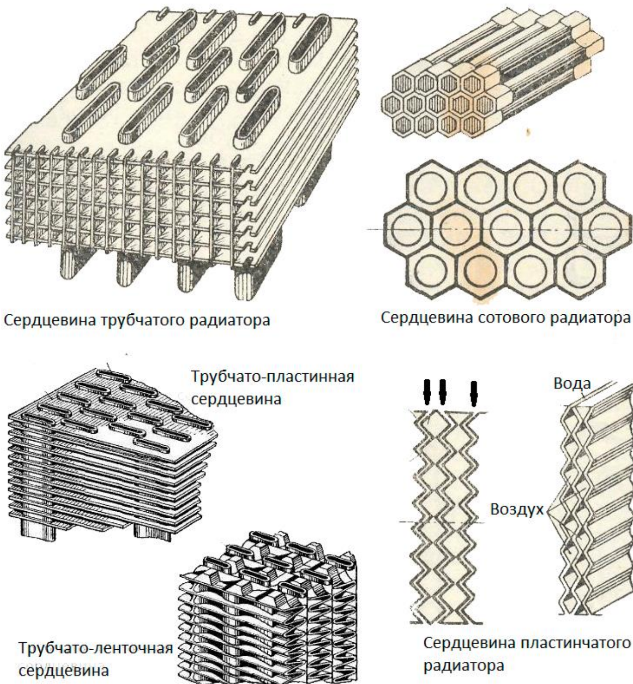
Рисунок 1.26 – Виды сердцевин радиатора
