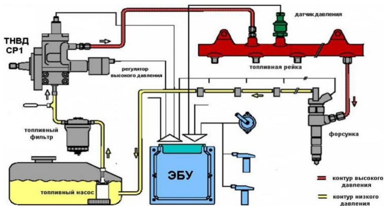
Рисунок 1.9 – Система впрыска топлива дизельного двигателя
