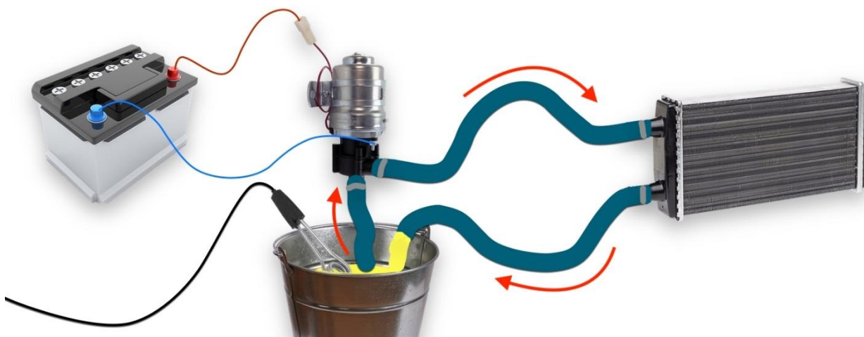
Рисунок 1.31 – Химическая чистка радиатора
