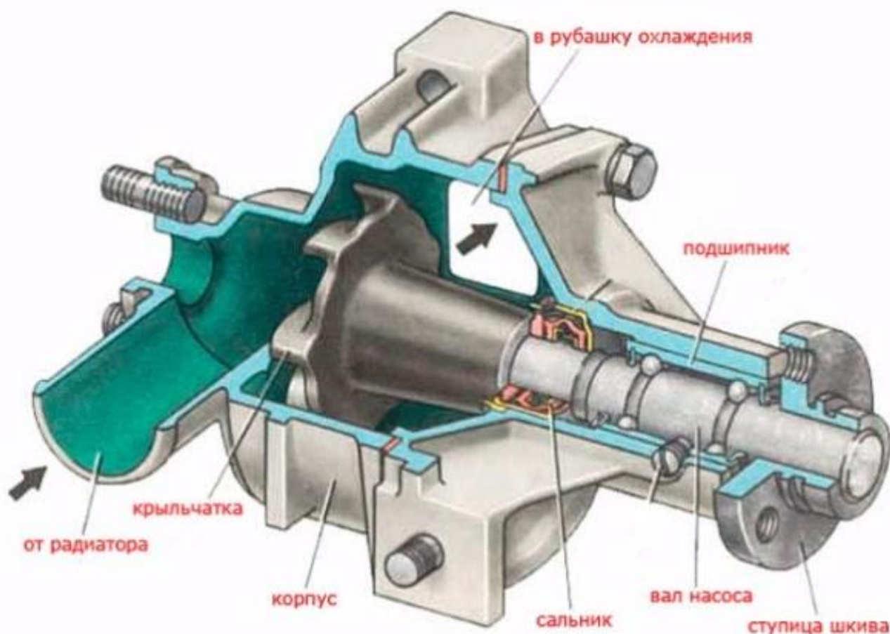
Рисунок 1.20 – Водяной насос системы охлаждения автомобиля
