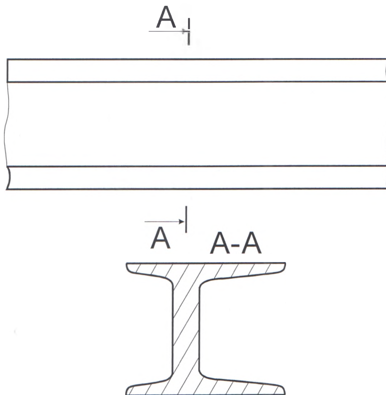
Рисунок 5.6 – Вынесенные сечения
