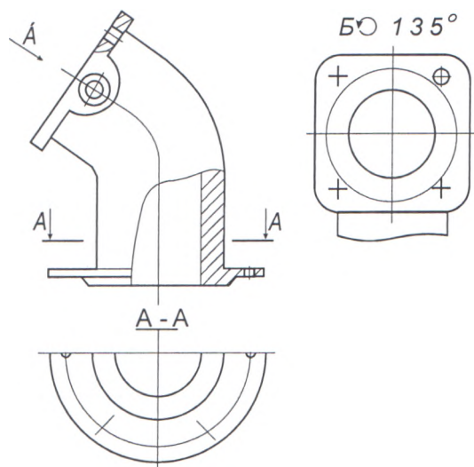
Рисунок 5.2 – Изображение на чертежах дополнительных видов
