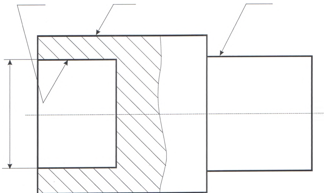
Рисунок 5.22 – Изображение на чертежах линий-выносок
