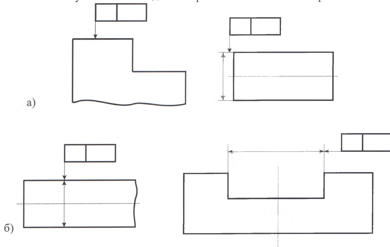
Рисунок 5.11 – Виды соединения рамки с поверхностью
