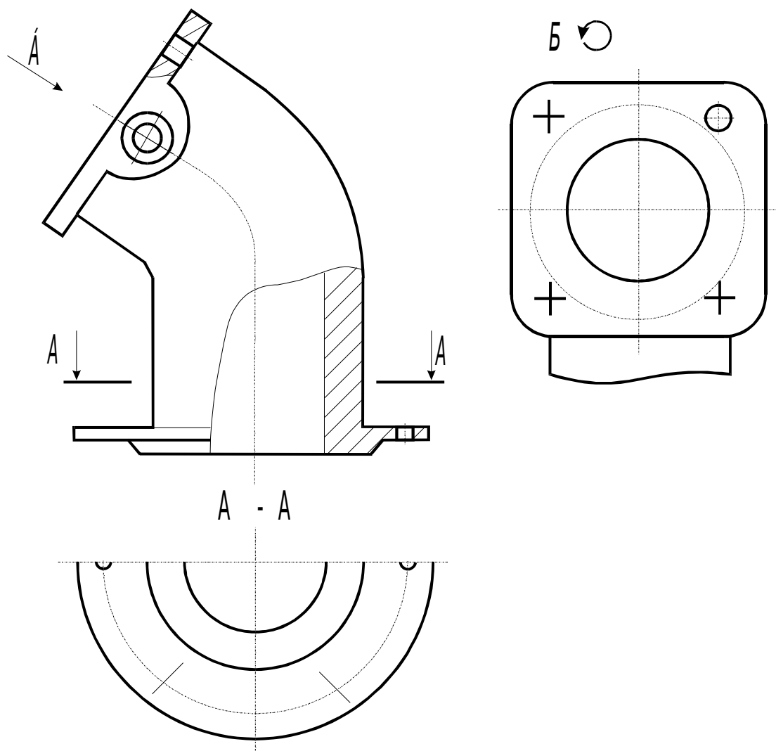
Рисунок 5.2 – Изображение на чертежах дополнительных видов
