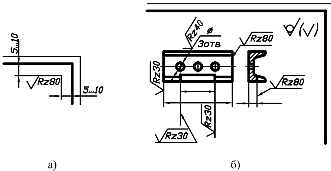
Рисунок 5.16 – Обозначение одинаковой шероховатости
