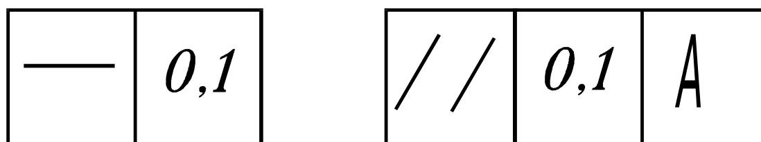
Рисунок 5.9 – Обозначение данных о допусках формы и расположения поверхностей
