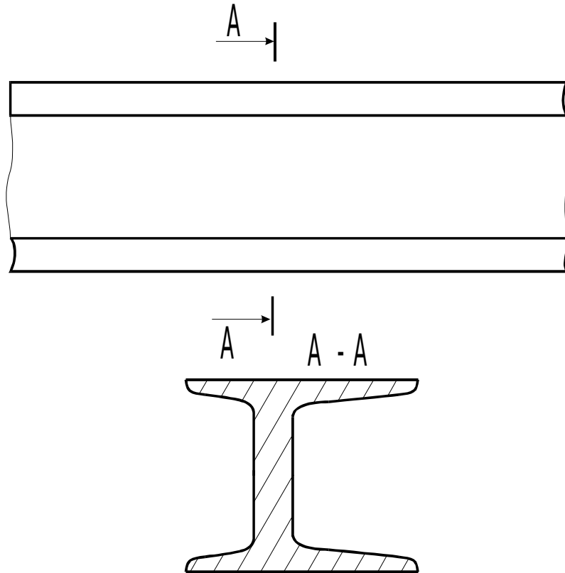
Рисунок 5.6 – Вынесенные сечения
