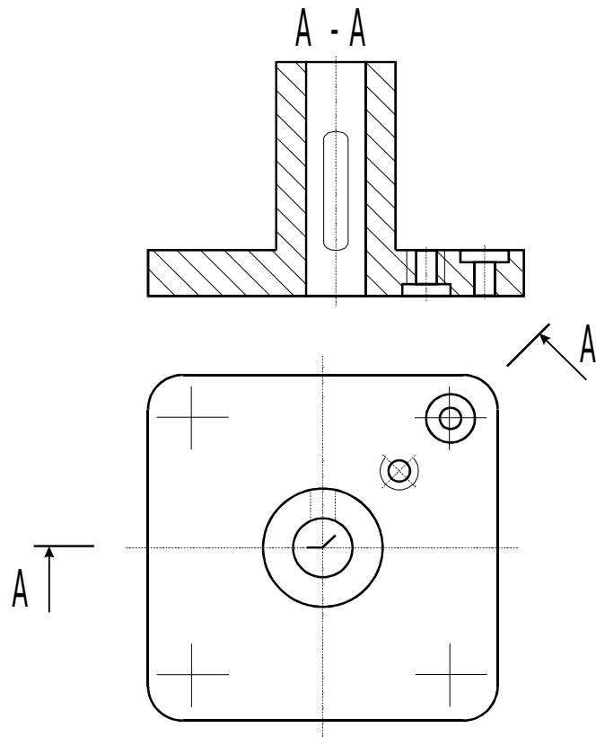
Рисунок 6.4 – Изображение разрезов и секущей линии на чертежах
