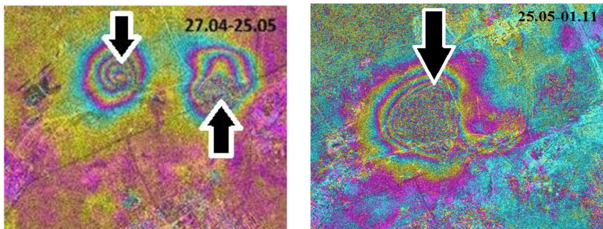
8-сурет – «Саранская» шахтасының маңындағы дифференциалды интерферограмма
