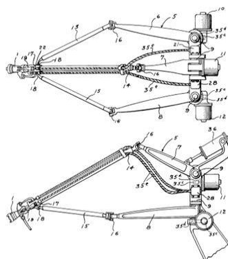
2 - сурет – 1938 жылғы Уиллард Л.В. Поллардтің манипуляторы
