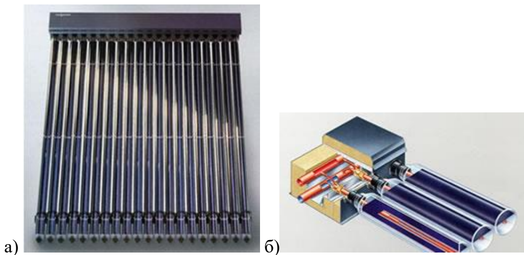
1.3-сурет – Виссман фирмасының вакуумды коллекторы: а) жалпы түрі, б) монтажды схемасы
