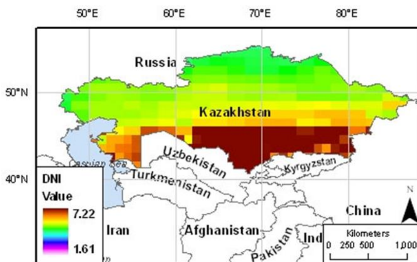
2.1-сурет – Күн сәулесінің тік сәулеленуі
