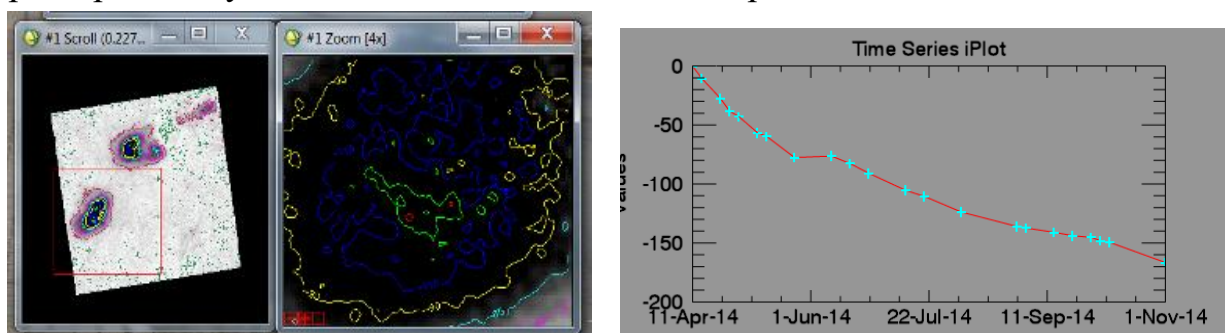
9-сурет – «Саранская» шахтасында барлық байқау мерзімінде жасалған ғарыштық суреттер бойынша салынған изосызықтар, «Саранская» шахтасының жұмыстар жүргізу аймағында жер бетінің шөгуінің максималды шамасы
