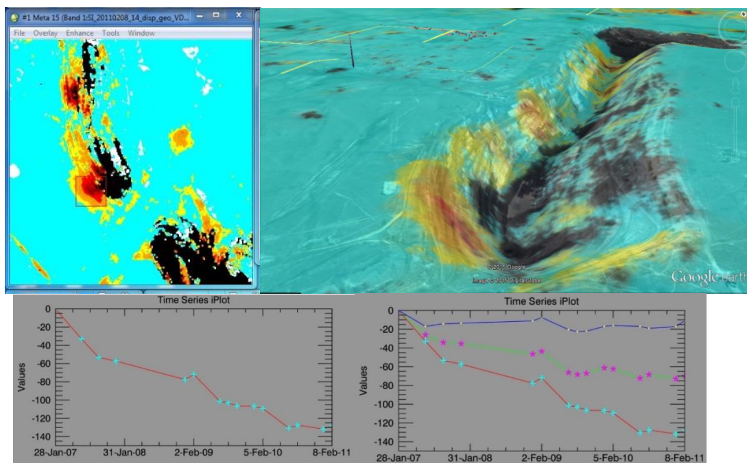
10-сурет – «Северный» разрезінің оңтүстік-батыс аймағындағы жер бетінің шөгуінің максималды шамасы
