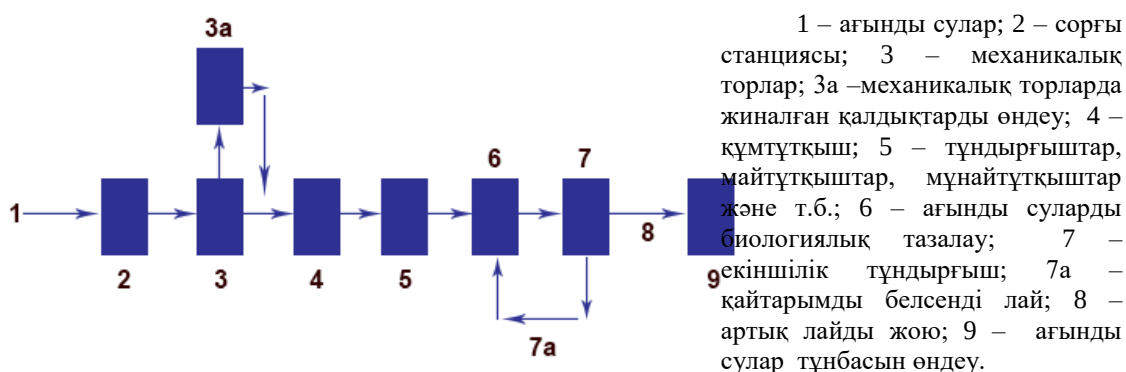
2-сурет - Ағынды суларды тазартудың жалпыланған жүйесі
