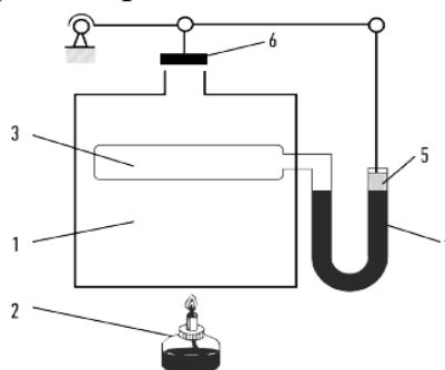
5 - сурет – Дреббель термостаты
